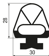
TIPO B2N
